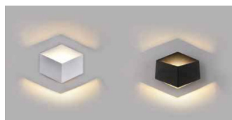
8344, 8346 fali lámpa 3W, 300lm, 230V, 3000K, fehér és fekete színben, IP20, 220 x 200 x 80 mm
