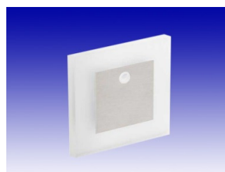
APUS LED PIR falba süllyeszthető lámpa 0,8W, 12V, 13lm, 3000K, IP20, 75 x 75 x 23 mm, mozgásérzékelővel
