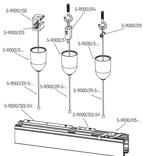
Egyedi kiegészítők: lehetséges kombinációk mennyezeti beállítókkal / Single accessories: possible combinations with ceiling regulation
