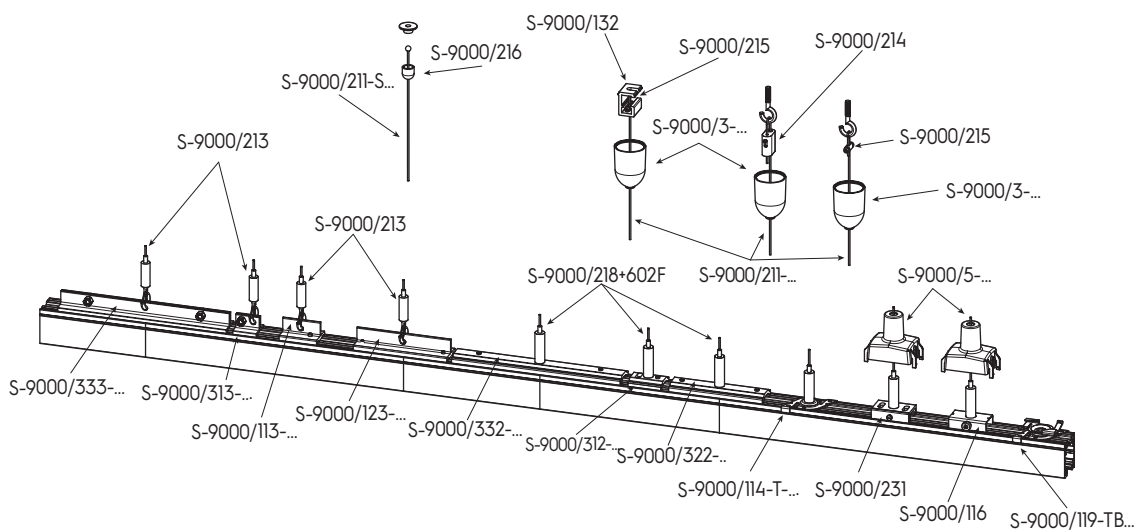
Egyedi kiegészítők: lehetséges kombinációk sín-beállítókkal / Single accessories: possible combinations with track regulation
